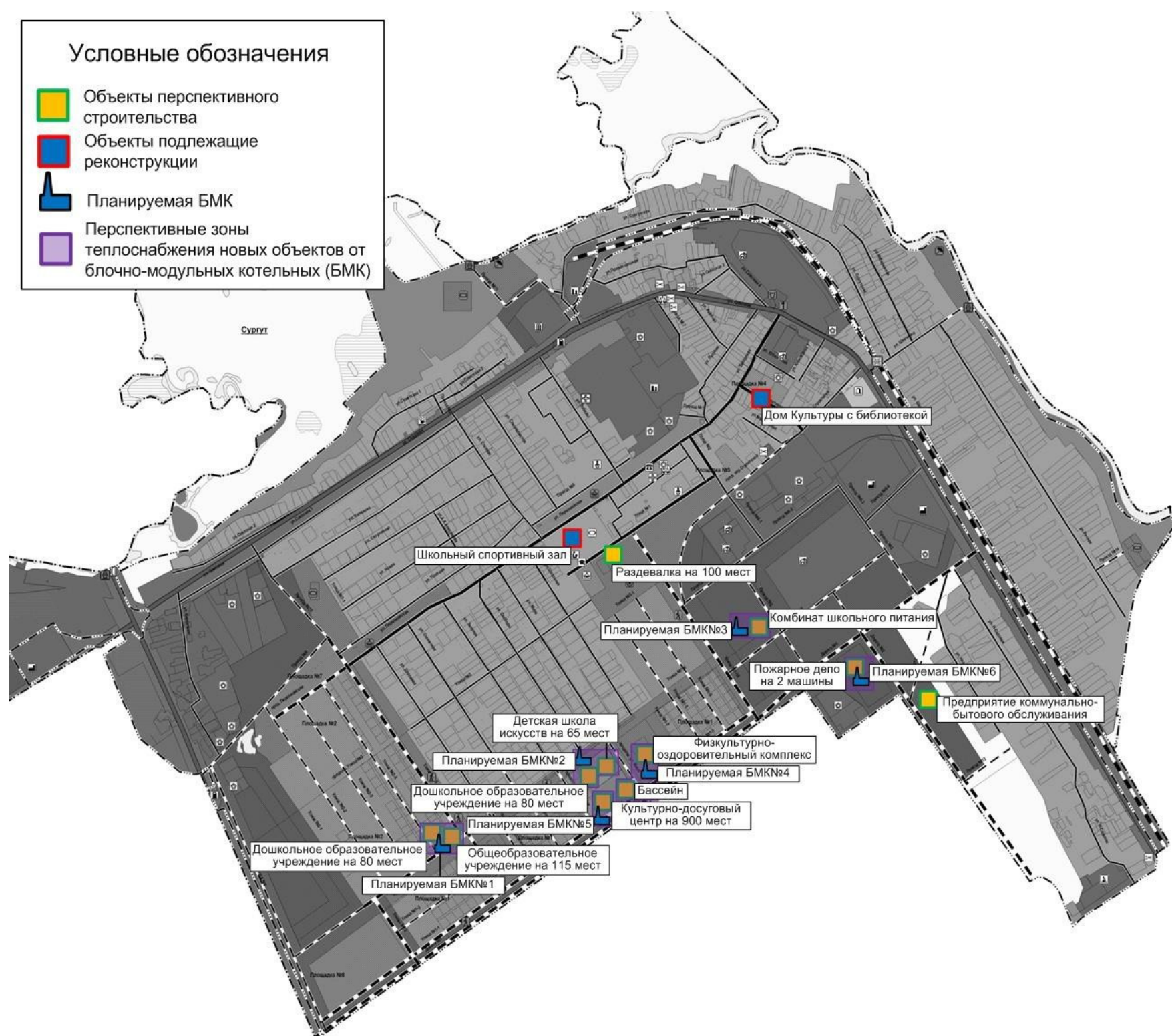
Рисунок 2.1.2 – Перспективная зона теплоснабжения планируемого блочно-модульного источника тепловой энергии, действующего на территории п. Сургут
